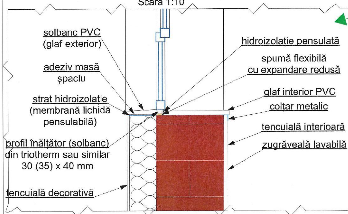
Detaliu de execuție - montaj tâmplărie exterioară - - secțiune - ferestre - Scara 1:10
