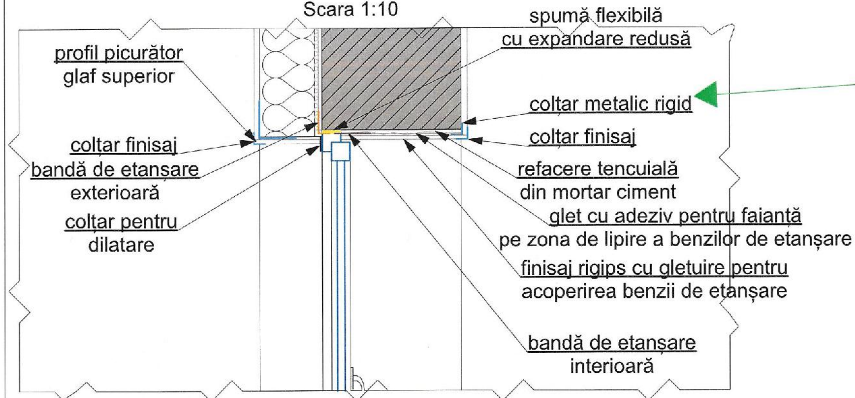
Detaliu de execuție - montaj tâmplărie exterioară - - secțiune - ferestre - Scara 1:10
