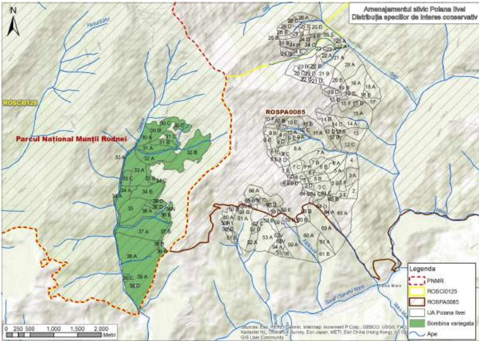
Distribuția potențială a speciei Bombina variegata
